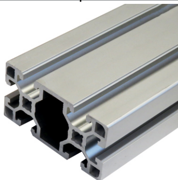
SIGMA 4001B profil 90x45 al sm
