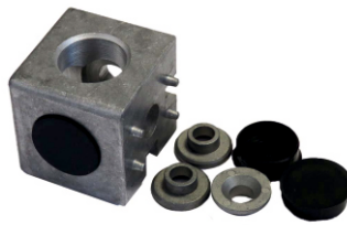
SIGMA kocka 3 kraka 45x45 zamak
