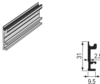
PVD TS-1700 nosač 1720 AL (PVS)
