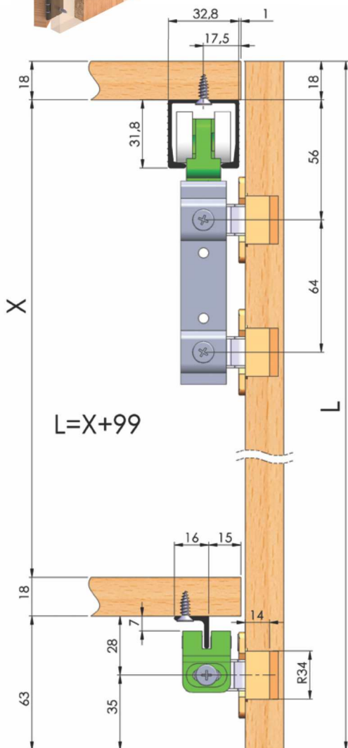
Šema postavke klizne šarke kada se klizna šina nalazi ispod korpusa
