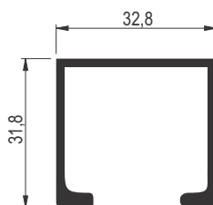
AL - 03 Gornja šina
