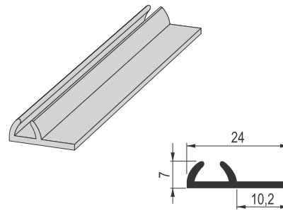
SM 45 šina 1k L-91 AL SM
