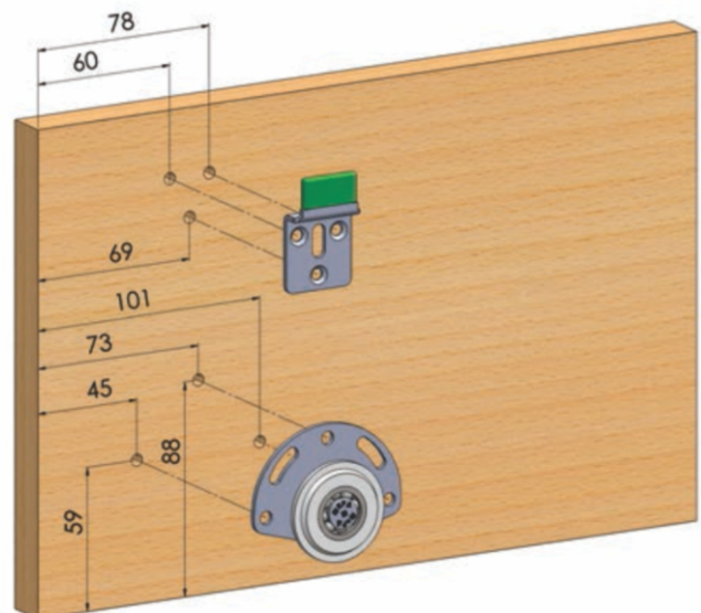
Prikaz šeme postavke mehanizma SM 37 na plakarska vrata
