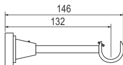
GH nosač jednokanalne garnišne
