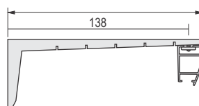
AL nosači za PRINCE garnišne (1k i 2k)
