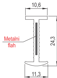
GP 04 E kraj za fleks. garnišnu
