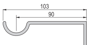
Metalni nosač za Eta garnišne
