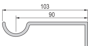
Metalni nosač za Čarli garnišne
