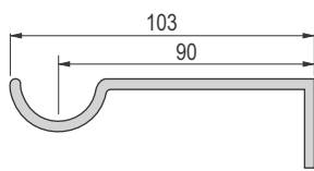
Metalni nosač za Harmony garnišne
