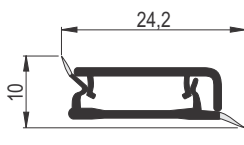
Horizontalno postavljanje
