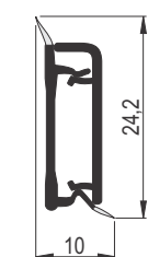
Vertikalno postavljanje
