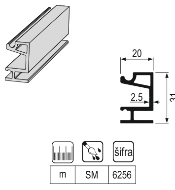
PVD TS-1700 nosač 1710 AL (PVS)
